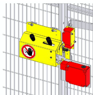
Safe Lock mit Notaus
